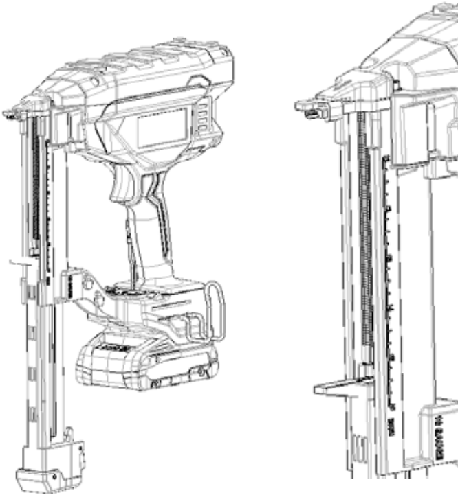
Abbildung 4: Gerät entladen
